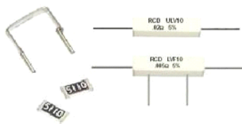
低阻电阻
